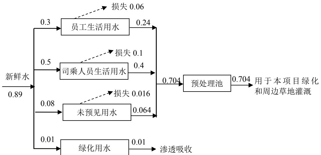
图 2-1 项目最大水量平衡见图 (m 3 /d)
